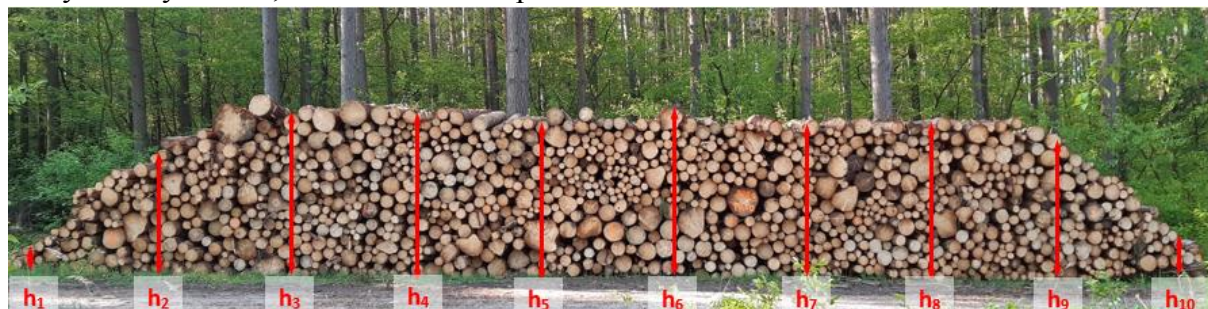
Ryc. 12. Pomiar wysokości stosu. Na czoło stosu naniesiono siatkę pomiarową, w której odległości pomiarami wynoszą 2 m
